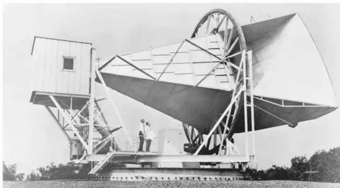
▲ Antena, za pomocą której odkryto mikrofalowe promieniowanie tła (jego mapę widziałeś na s. 202)
