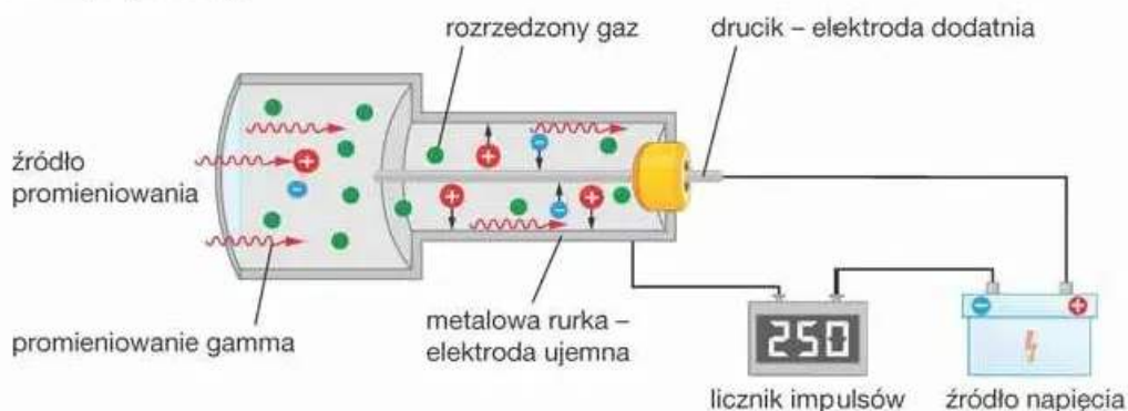
▲ Schemat licznika Geigera–Müllera
