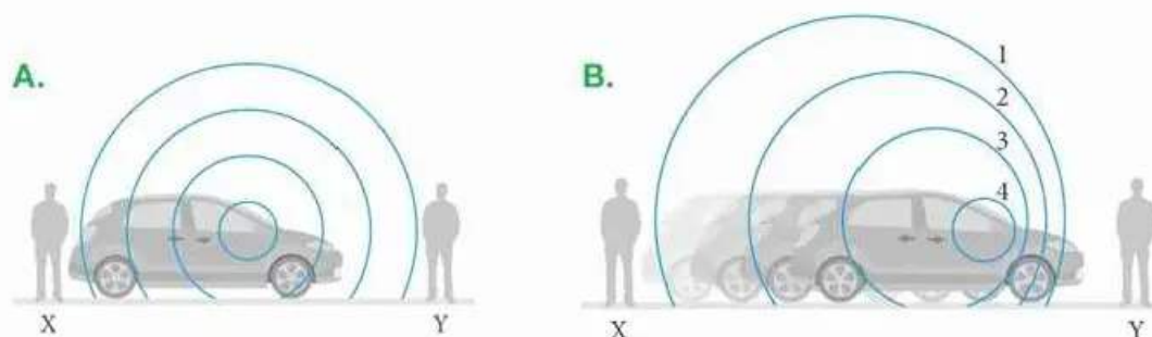
▲ Samochód z włączonym klaksonem: w spoczynku (A), w ruchu (B)
