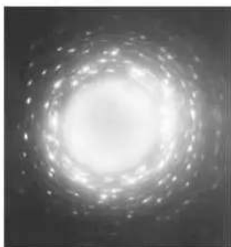
▲ Obraz interferencyjny powstały po przepuszczeniu wiązki elektronów przez kryształ tlenku talu (A) oraz schematyczny rysunek ułożenia atomów w tym kryształach (B)
