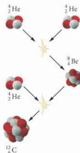
▲ Schemat reakcji przemiany helu w węgiel
