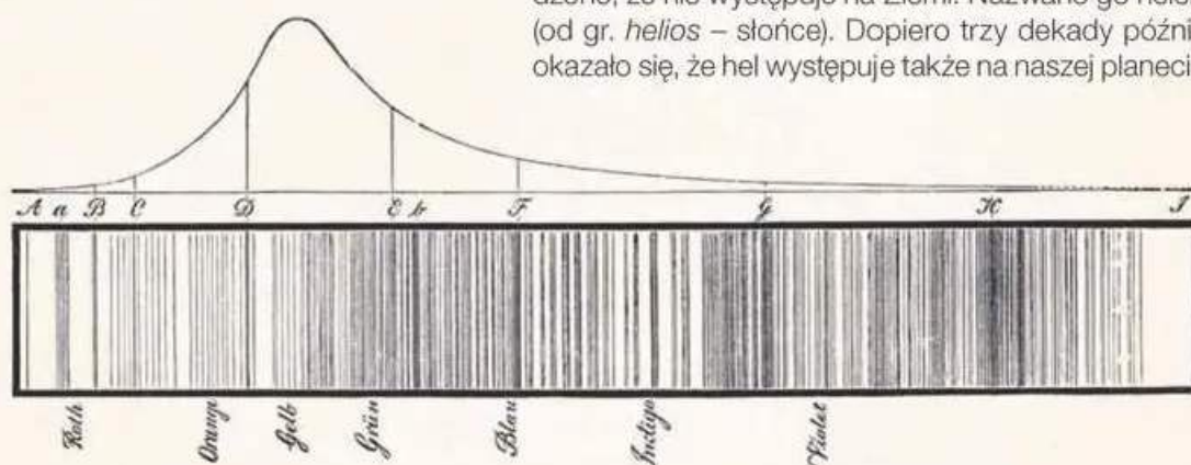
▲ Rysunek sporządzony przez Fraunhofera przedstawiający widmo słoneczne
