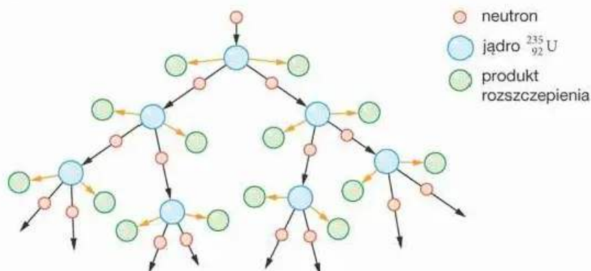
▲ Reakcja łańcuchowa zachodząca w bryle uranu ^{235}_{92}\text{U} (bez zachowania skali). Czarne strzałki przedstawiają tory ruchu neutronów, które spowodowały rozszczepienie kolejnych jąder uranu
