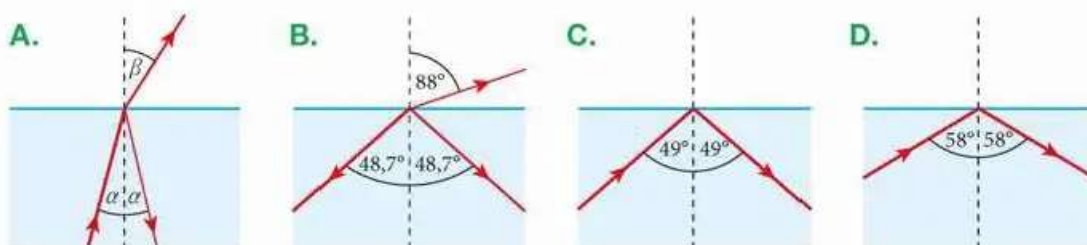
▲ Odbicie wewnętrzne: częściowe (A i B), całkowite (C i D)
