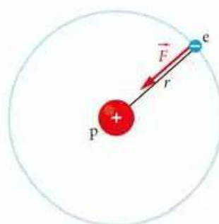
▲ Siła działająca na elektron w atomie Bohra
