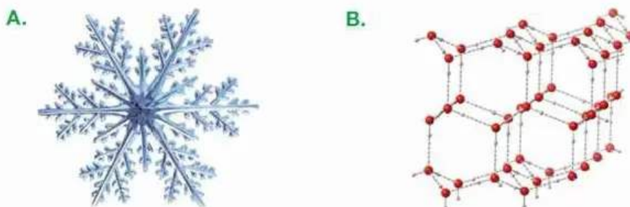
▲ Kształt płatka śniegu (A) wynika z układu atomów tlenu (czerwone) i wodoru (szare) w kryształach lodu (B)
