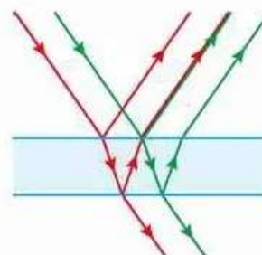
▲ Interferencja na błonie bańki mydlanej; kolory promieni służą tylko ich rozróżnieniu na rysunku, w rzeczywistości są to promienie światła białego
