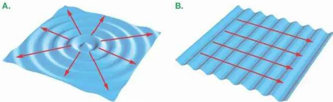
▲ Fale koliste (A) i płaskie (B) na wodzie. Czerwone linie to promienie fali
