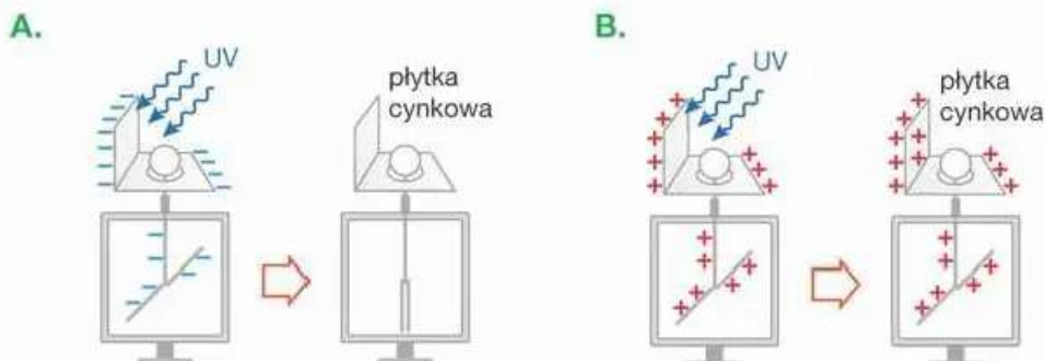
▲ Ujemnie naładowany elektroskop (A) rozładowuje się pod wpływem promieniowania ultrafioletowego (UV). Dodatnio naładowany elektroskop (B) nie ulega rozładowaniu
