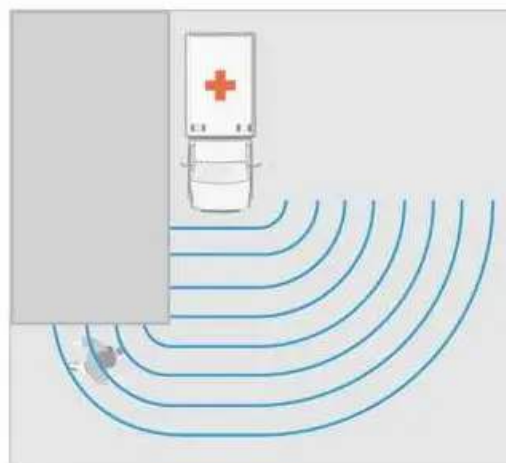
▲ Ugięcie fal dźwiękowych na krawędzi budynku
