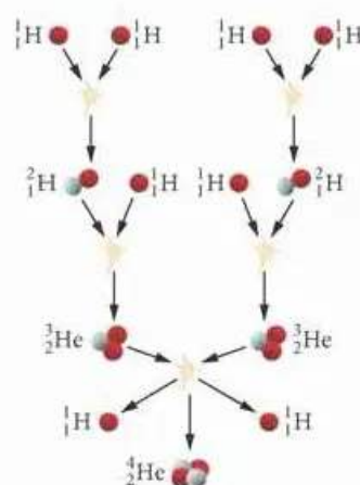
▲ Uproszczony schemat syntezy wodoru w hel
