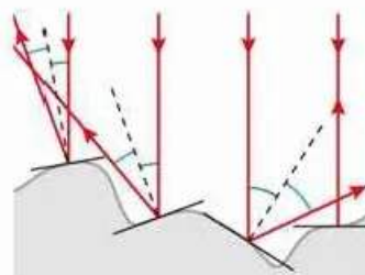
▲ Rozproszenie po odbiciu od nieregularnej powierzchni. Dla każdego z promieni zaznaczono styczną do powierzchni, linię do niej prostopadłą oraz kąt padania i kąt odbicia
