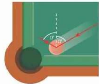
▲ Prawo odbicia dla kul bilardowych
