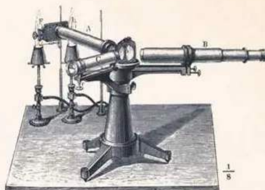
▲ Spektroskop zbudowany przez Fraunhofera
