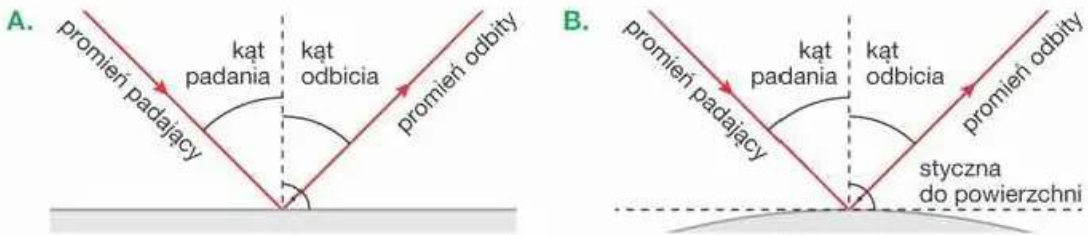
▲ Kąt padania i kąt odbicia od płaszczyzny (A) i od zakrzywionej powierzchni (B)
