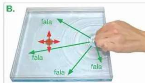
▲ Porównanie ruchu fali i ruchu ciała na wodzie
