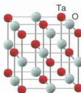
▲ Obraz interferencyjny powstały po przepuszczeniu wiązki elektronów przez kryształ tlenku talu (A) oraz schematyczny rysunek ułożenia atomów w tym kryształach (B)
