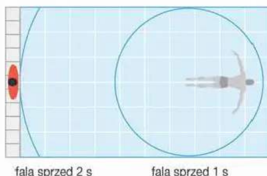
▲ Efekt Dopplera dla fal na wodzie - źródło oddala się do obserwatora
