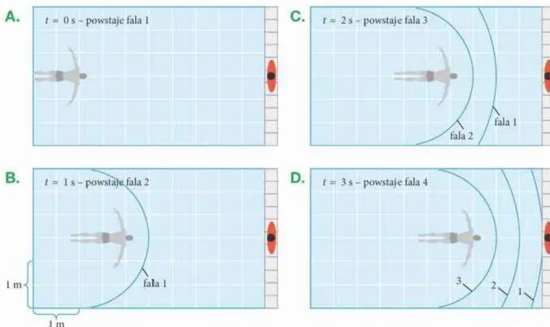
▲ Efekt Dopplera dla fal na wodzie – źródło zbliża się do obserwatora
