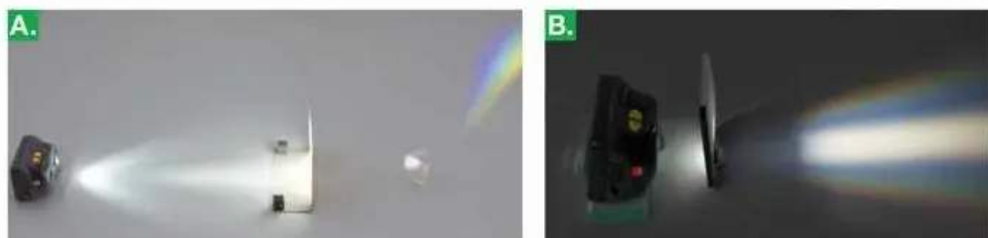
▲ Widmo światła białego po przejściu przez: pryzmat (A) i siatkę dyfrakcyjną (B)
