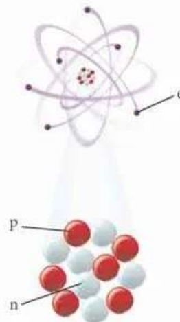
▲ Model atomu węgla i jego jądra, oznaczenia: e – elektron, p – proton, n – neutron
