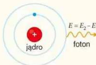
▲ Atom po emisji fotonu
