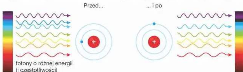
▲ Atom gazu pochłania tylko fotony o pewnej energii
