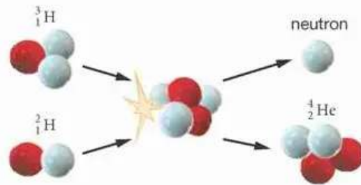
▲ Reakcja syntezy jąder trytu i deuteru
