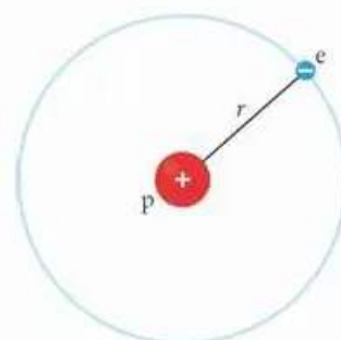
▲ Atom wodoru według Bohra
