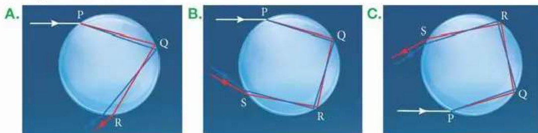
▲ Powstawanie drugiej (zewnętrznej) tęczy
