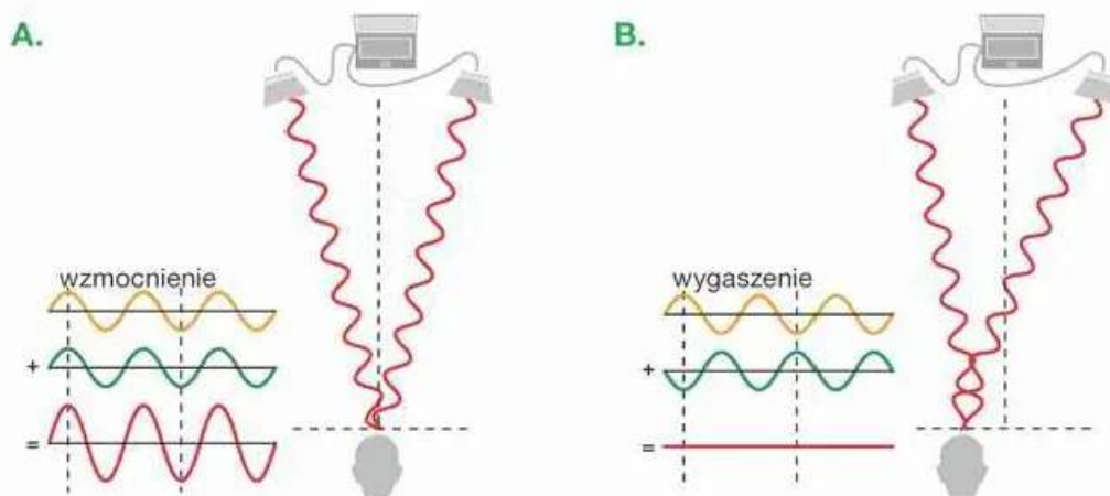
▲ Interferencja fal dźwiękowych: A. wzmocnienie fal, B. wygaszenie fal
