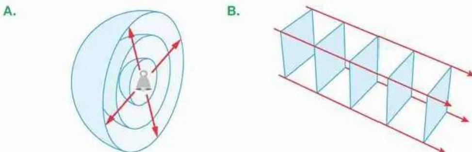
▲ Promienie i powierzchnie falowe: A. kulistej fali dźwiękowej, B. fali płaskiej w przestrzeni
