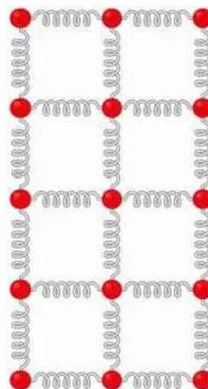
▲ Kulki połączone sprężynkami – model oddziaływań cząsteczek w ciele stałym
