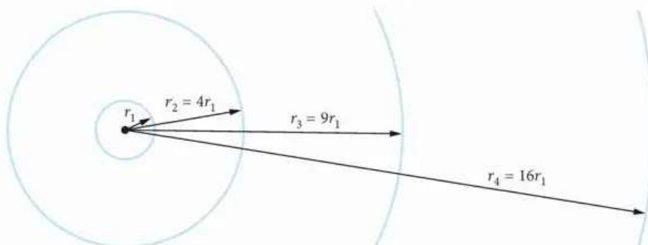
▲ Cztery pierwsze orbity atomu wodoru z zachowaniem proporcji odległości
