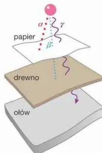
▲ Zasięg promieniowania alfa, beta i gamma
