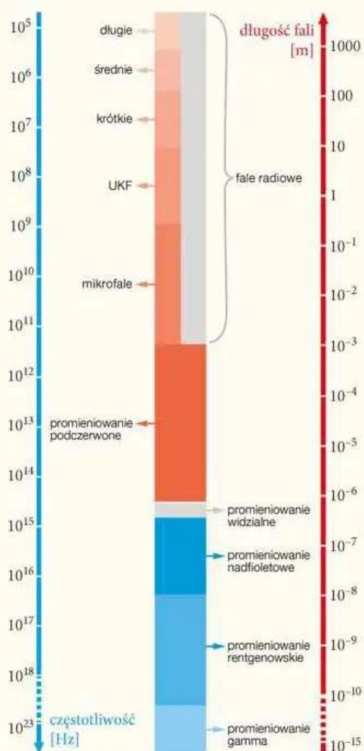
▲ Widmo fal elektromagnetycznych
