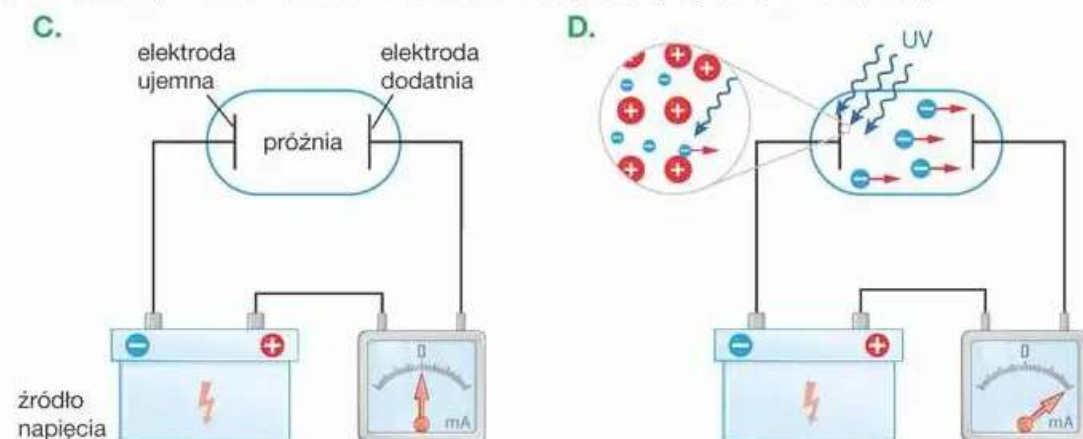
▲ Prąd nie płynie (C). Światło wybija elektrony z elektrody ujemnej i prąd płynie (D)
