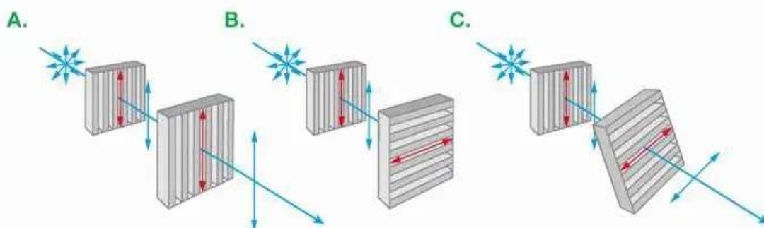
▲ Przejście światła przez dwa kolejne polaryzatory
