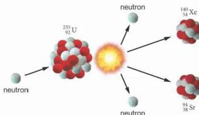
▲ Rozszczepienie jądra uranu
