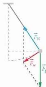
▲ Sytuacja tuż po puszczeniu wahadła
