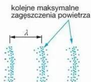
▲ Długość fali dźwiękowej
