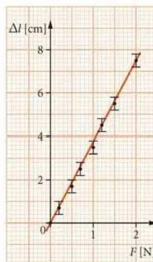
▲ Wykres zależności wydłużenia sprężyny od siły rozciągającej
